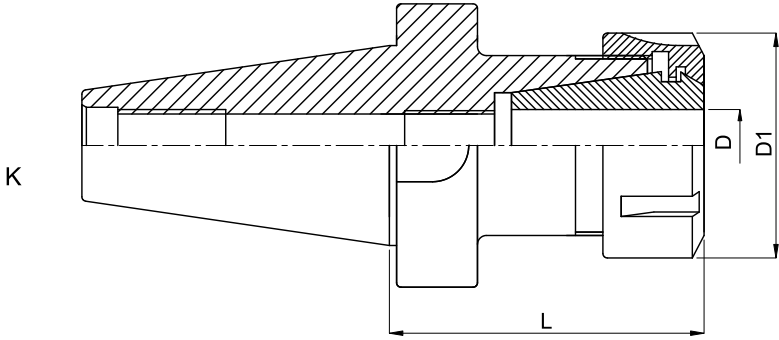
DIN 2080 CONO TRONCO
